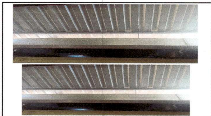
Foto 10: Sustitución de canal de metal por canales de lamina aluzinc calibre 24 con sujetadores en corredores. Módulo 7
